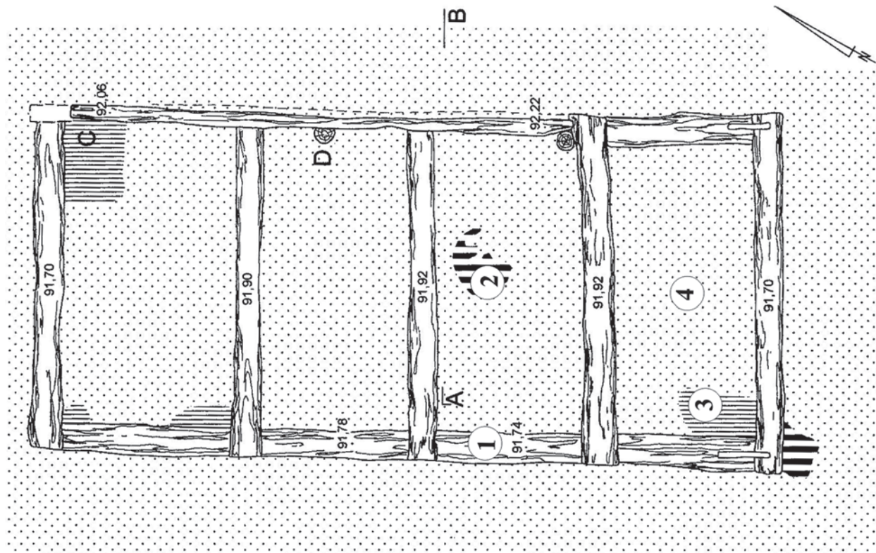
Ryc. 17. Bolimów, stan. 9, gm. loco, woj. łódzkie. Obiekt 48 – schron drewniano-ziemny. 1: drewno; 2: spalone drewno; 3: ciemnobrunatna próchnica; 4: żółty piasek
