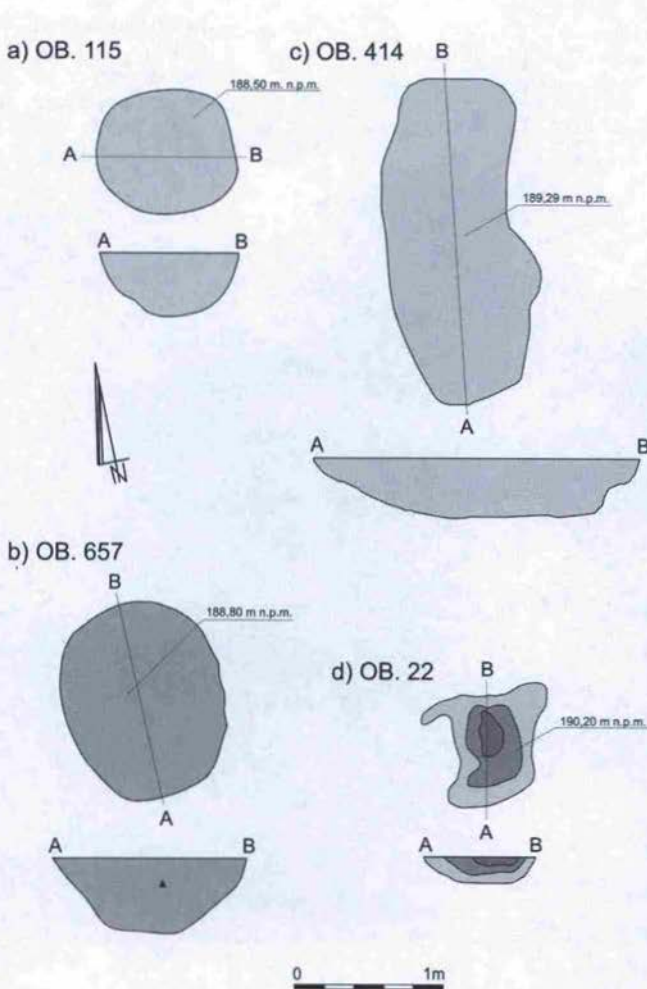
Ryc. 5. Nowa Wieś 2/4. Obiekty gospodarcze: a – nr 115, b – nr 657, c – nr 414; palenisko: d – nr 22. Rys. J. Domańska, K. Czarniak, R. Szwed
