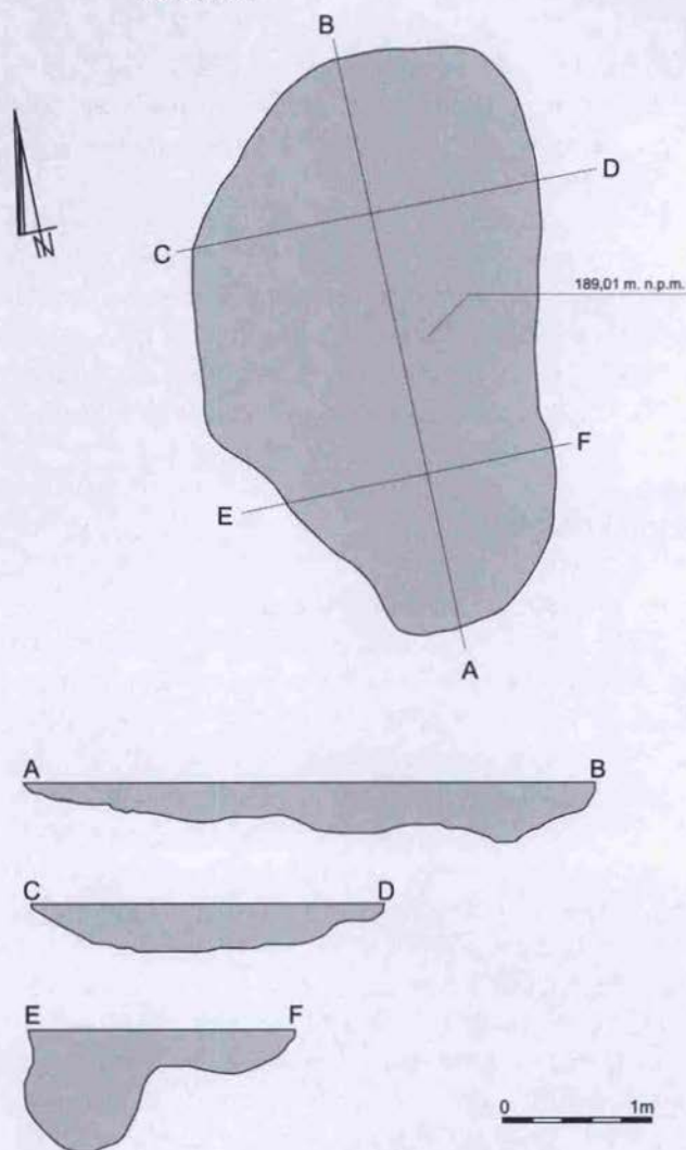
Ryc. 4. Nowa Wieś 2/4. Obiekt mieszkalny nr 442. Rys. R. Szwed
