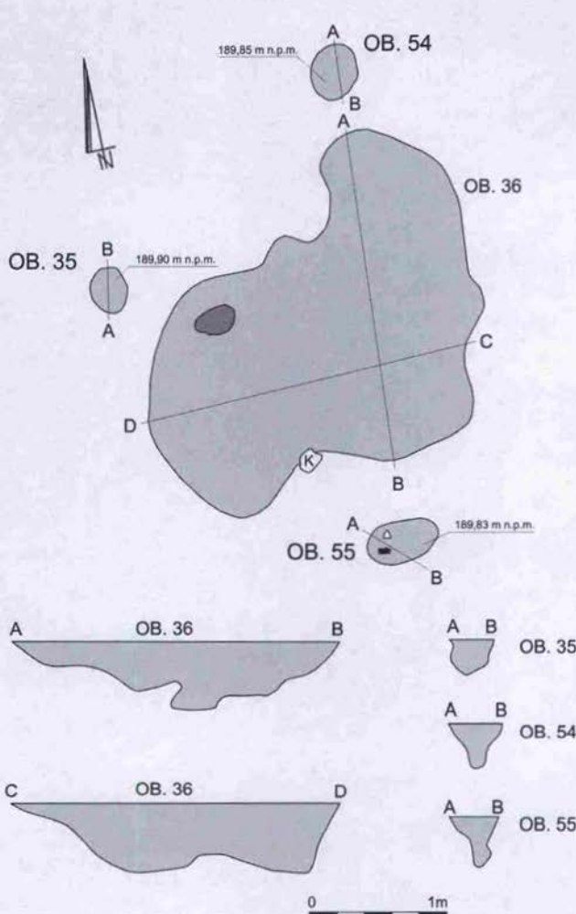
Ryc. 6. Nowa Wieś 2/4. Obiekt nr 36 i towarzyszące mu obiekty posłupowe nr 35, 54, 55. Rys. J. Domańska
