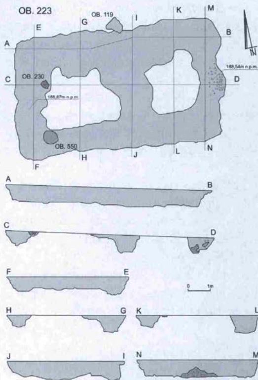
Ryc. 7. Nowa Wieś 2/4. Obiekt kultowy nr 223. Rys. J. Domańska, P. Madera, R. Szwed, K. Ślipko-Jastrzębska
