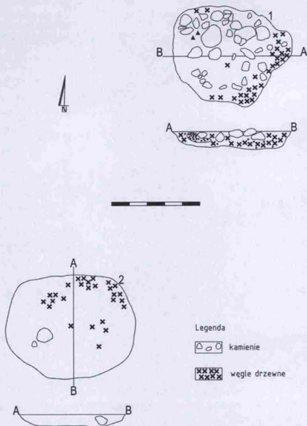
Ryc. 5. Przesieczany 6, gm. Zgorzelec. Rzuty poziome i przekroje obiektów nr 1 i 2 – palenisk (rys. J. Baron).
