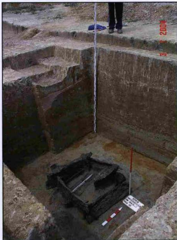
Ryc. 4. Stanisławice, stan. 9. Elementy konstrukcji studni – zbliżenie (fot. T. Rodak).
