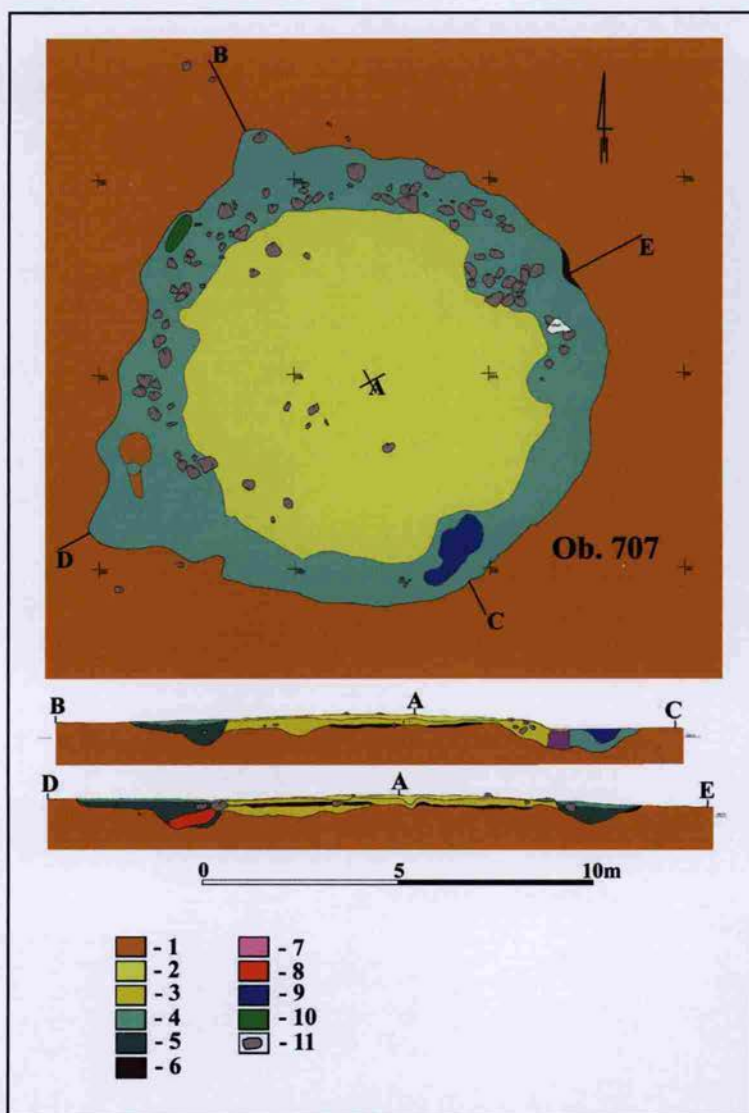
Ryc. 3 Jagłowice stan. 1, pow. Żary. Rzut poziomy i przekroje obiektu 707 (kurhanu L): 1 – jasnożółta próchnica przemieszana z ciemnożółtym piaskiem w układzie różnoplamistym; 2 – jasnożółty piasek przemieszany w układzie drobnoplamistym z ciemnoszarą próchnicą, drobne węgle drzewne; 3 – jasnożółty piasek w układzie jednolitym; 4 – brązowa próchnica w układzie jednolitym, niewielkie fragmenty węgla drzewnych; 5 – jasnobrązowa próchnica w układzie jednolitym, niewielkie fragmenty węgla drzewnych; 6 – ciemnożółty piasek przemieszany z gruboziarnistym żwirem i drobnymi kamieniami; 7 – brązowo-brunatna próchnica przemieszana z ciemnożółtym piaskiem w układzie średnioplamistym, drobne węgle drzewne; 8 – ciemnobrązowo-szara próchnica przemieszana w układzie drobnoplamistym z ciemnożółtym piaskiem; 9 – czarno-brązowa próchnica w układzie jednolitym, drobne węgle drzewne; 10 – ciemnoszaro-brązowa próchnica w układzie średnioplamistym z pomarańczowym i żółtym piaskiem; 11 – kamień.
