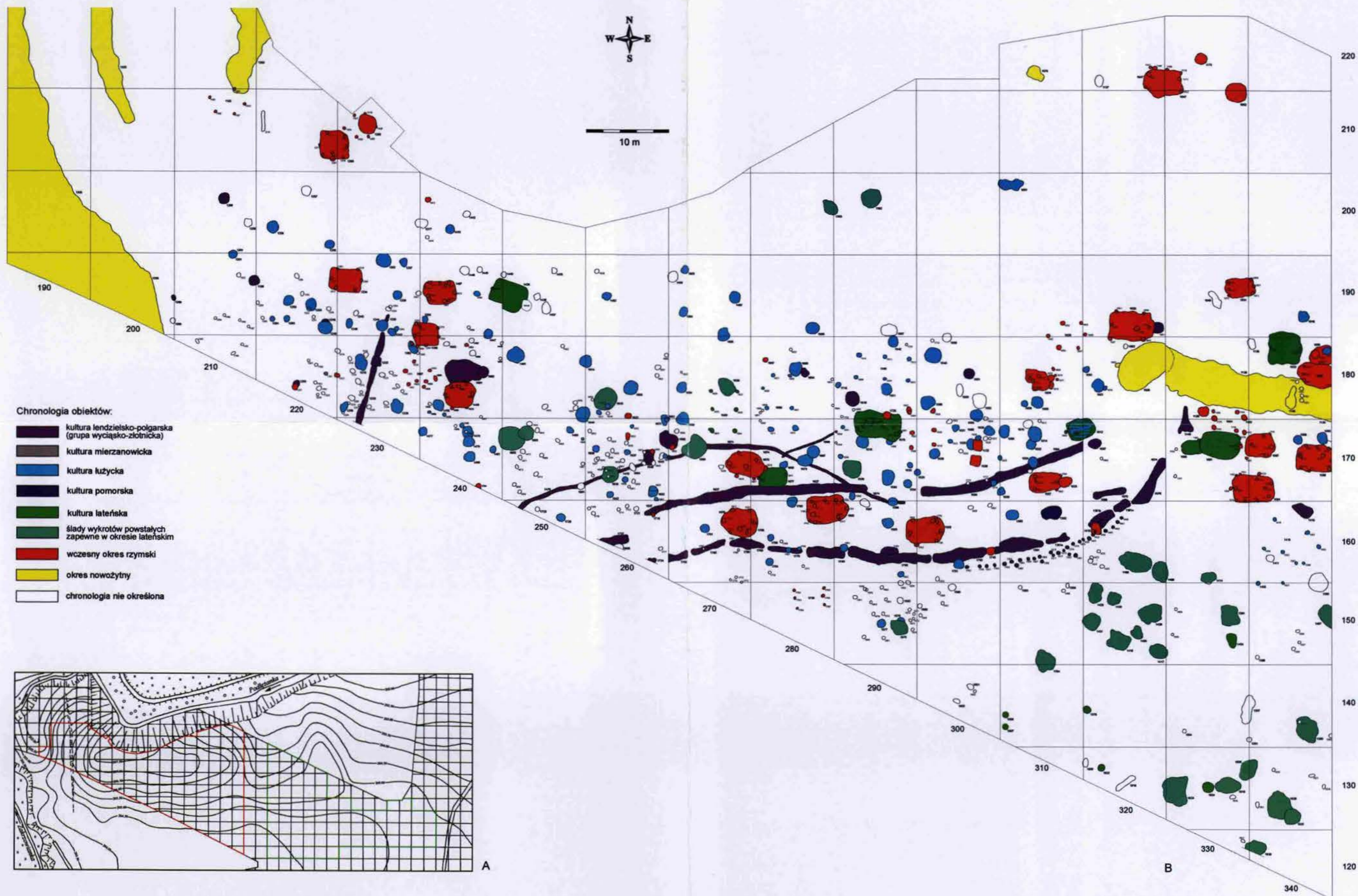
Ryc. 2. Podłęże, stan. 17. A: szkic sytuacyjny na podkładzie mapy hipsometrycznej z siatką arową naniesioną w obrębie pasa zajęcia autostrady; grupy arów przebadanych do końca 2004 r. zaznaczono kolorem czerwonym (ary w zachodniej części stanowiska; badania W. Machowskiego) i kolorem zielonym (ary we wschodniej części stanowiska; badania M. i K. Dzięgielewskich i R. Szczerby). B: plan części zachodniej stanowiska z zaznaczoną siatką arową i rozmieszczeniem obiektów archeologicznych (chronologia wg legendy) (stan badań do końca 2004 r.). Opr. K. Dzięgielewski.
