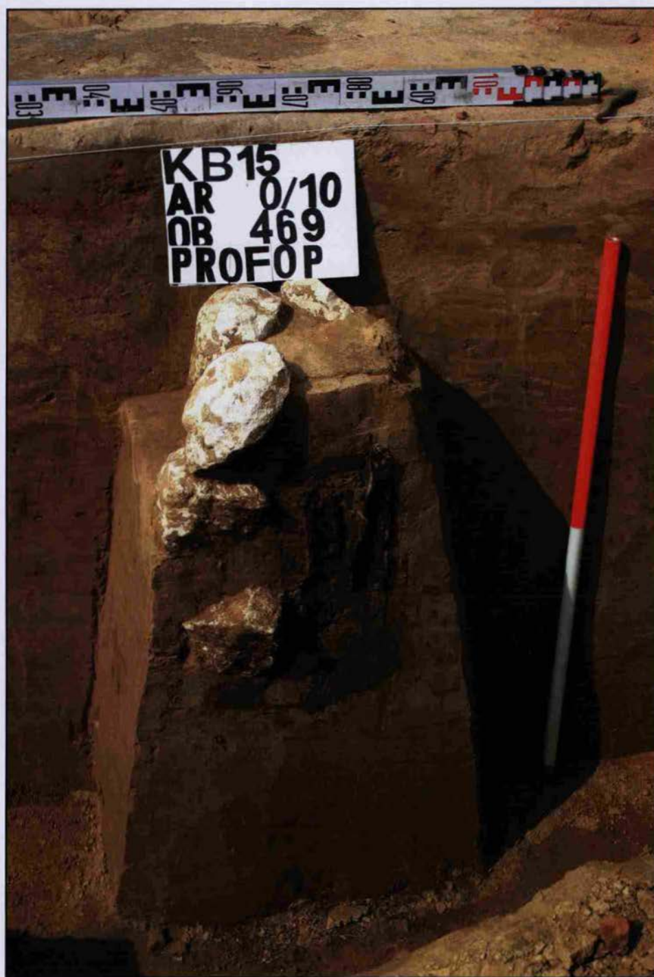
Ryc. 20. Częściowo zachowany słup drewniany obłożony kamieniami wapiennymi z chaty 243 ze stan. 15 w Krakowie-Bieżanowie.
