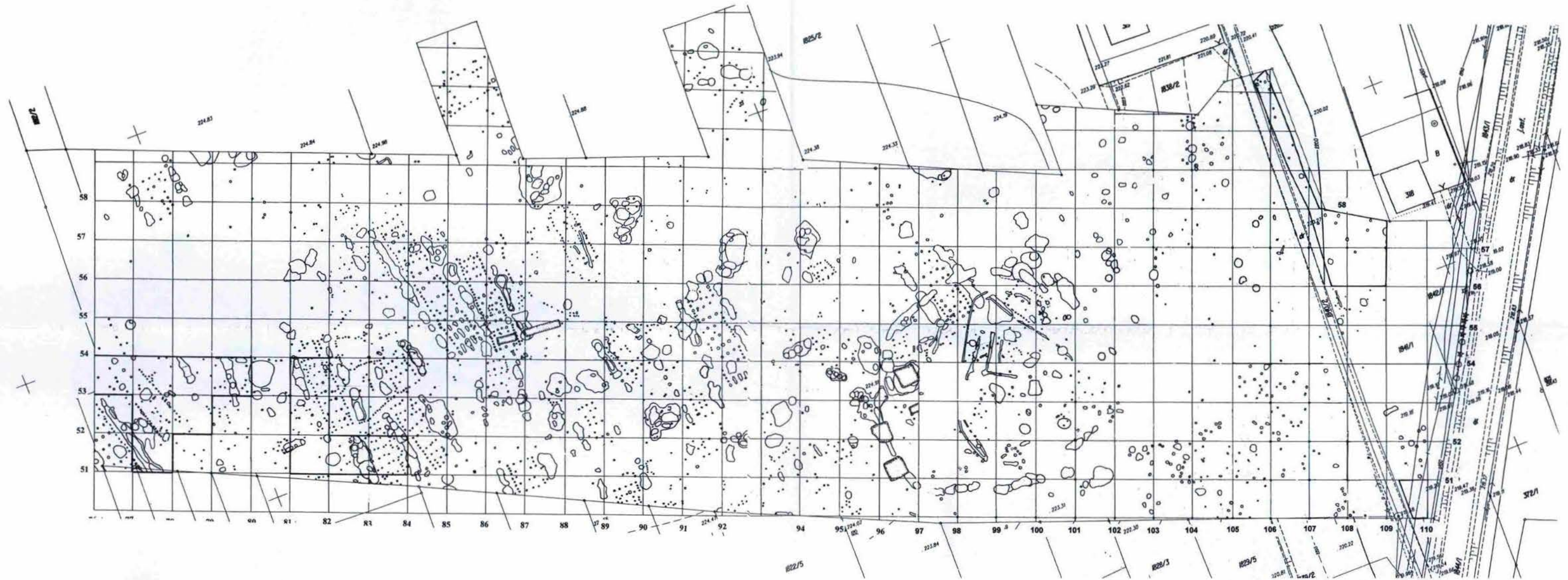
Ryc. 3. Długie domy kultury ceramiki wstęgowej rytej na tle innych wczesnoneolitycznych obiektów na stanowisku 12-13 w Targowisku (na podstawie siatki arowej; ryc. A. Golański).
