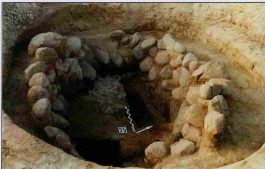
Ryc. 10. Stugocinek, st.1. Kamienny piec wapieniczny i garncarski. Fot. A. Krzyszowski
