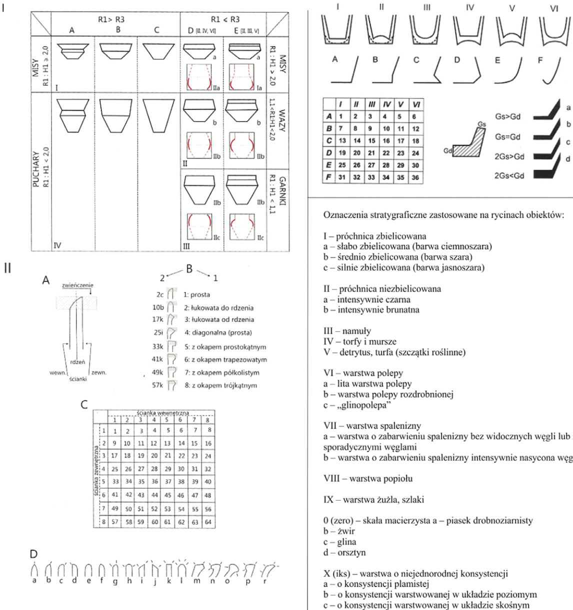
Ryc. 3 Klasyfikacja typów makromorfologicznych (wg Węgrzynowicz 1984 i Ignaczak 2016). Schemat systematyki krawędzi (wg Koško 1981) z uzupełnieniami (Ignaczak 2016, 60) oraz den (wg Czebreszuk 1996) z uzupełnieniami (Czebreszuk et al. 2006, 57)
